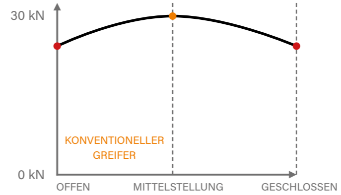
SCHLIESSKRAFTVERLAUF
